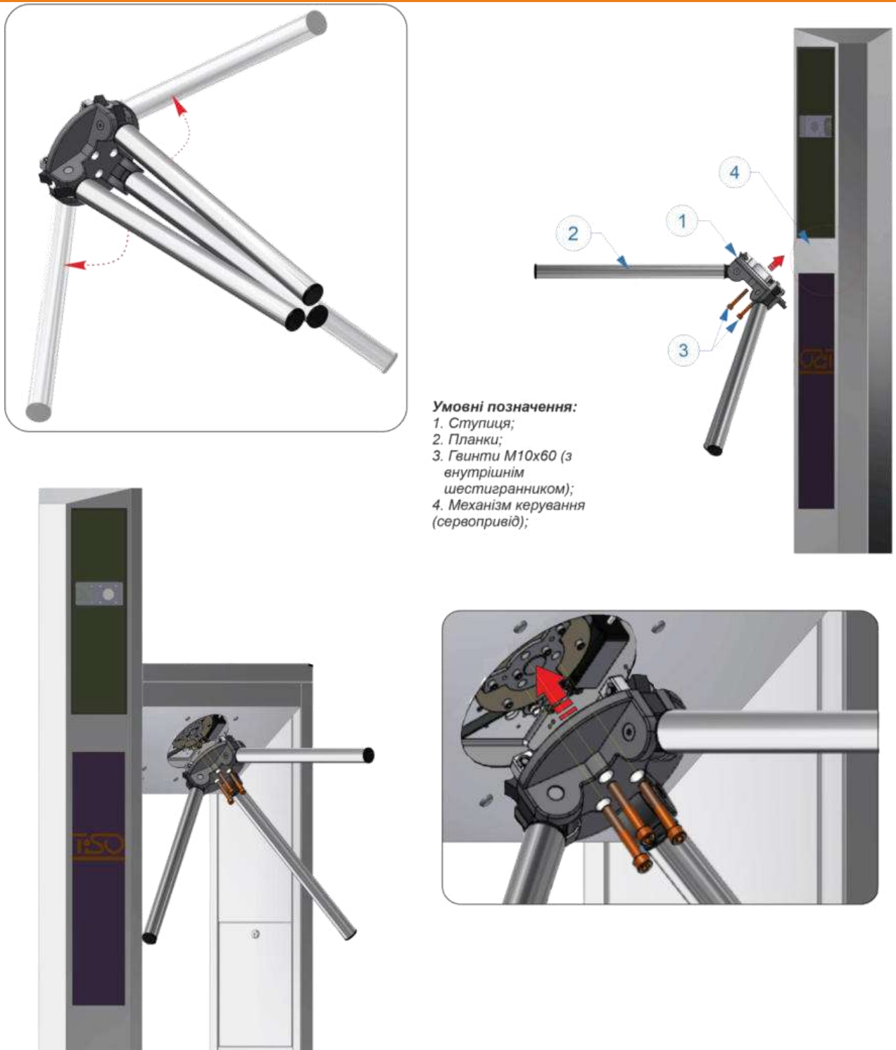
Рис. 13– Встановлення ступиці з планками в корпус турнікету-триподу
