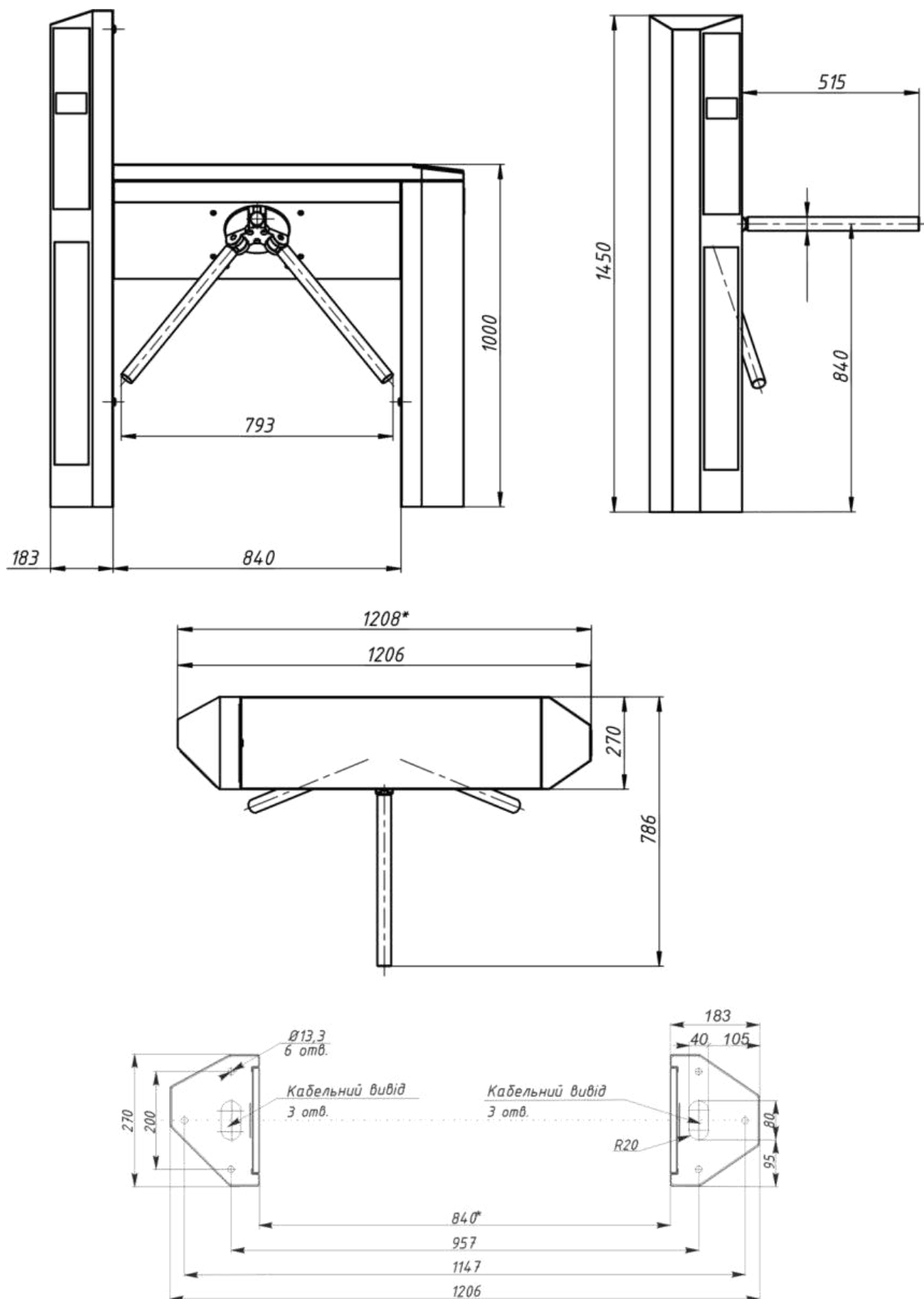
Додаток А.1. Монтажне креслення турнікету-триподу «TWIX ALL IN ONE- М»
