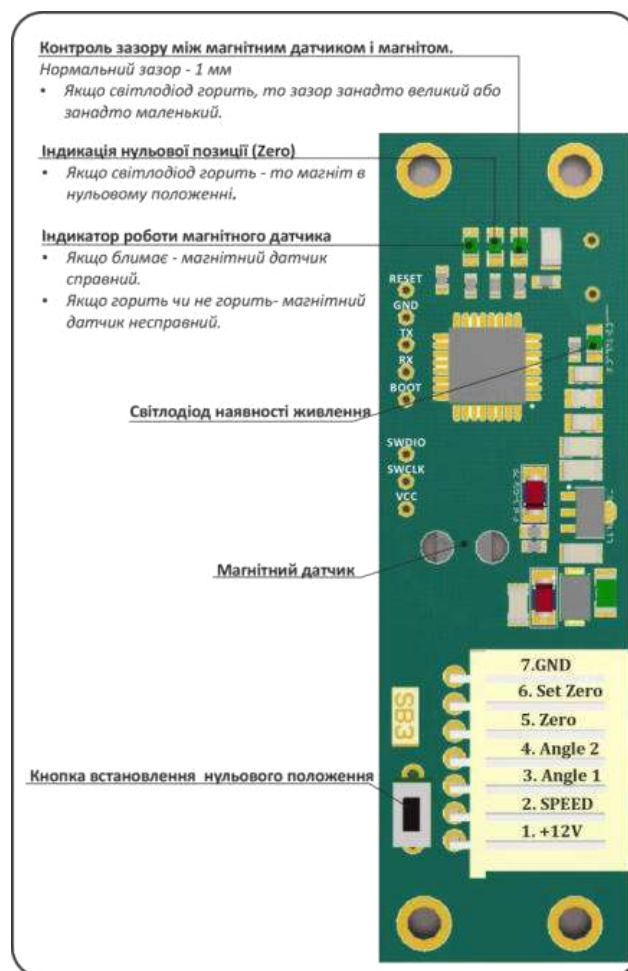
Рис. 18– Опис контролера магнітного датчика
