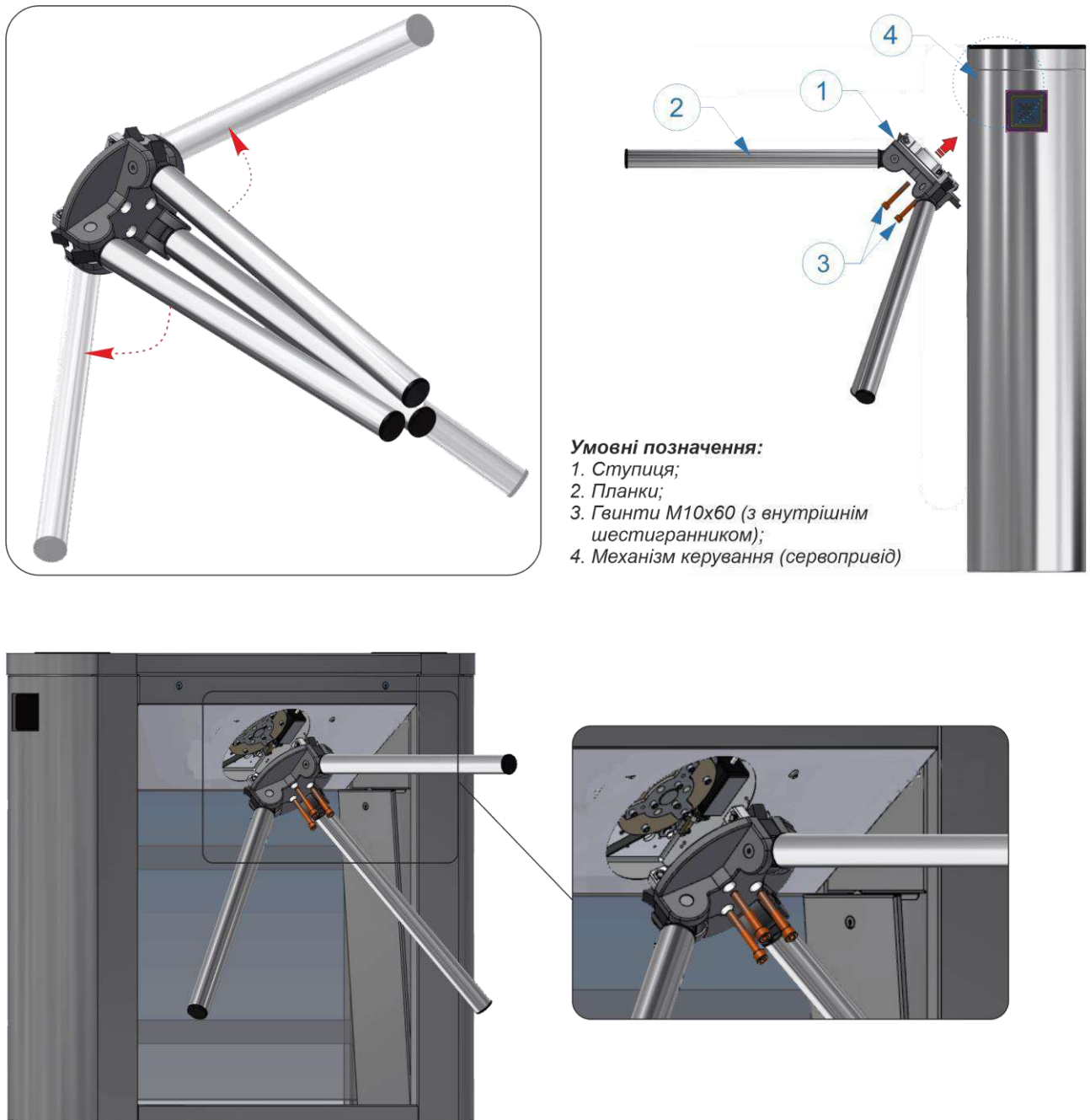
Рис. 14 – Встановлення ступиці з планками в корпус турнікету-триподу
